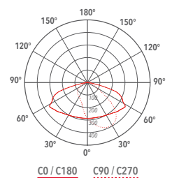
Strade extraurbane secondarie e urbane - centri storici
